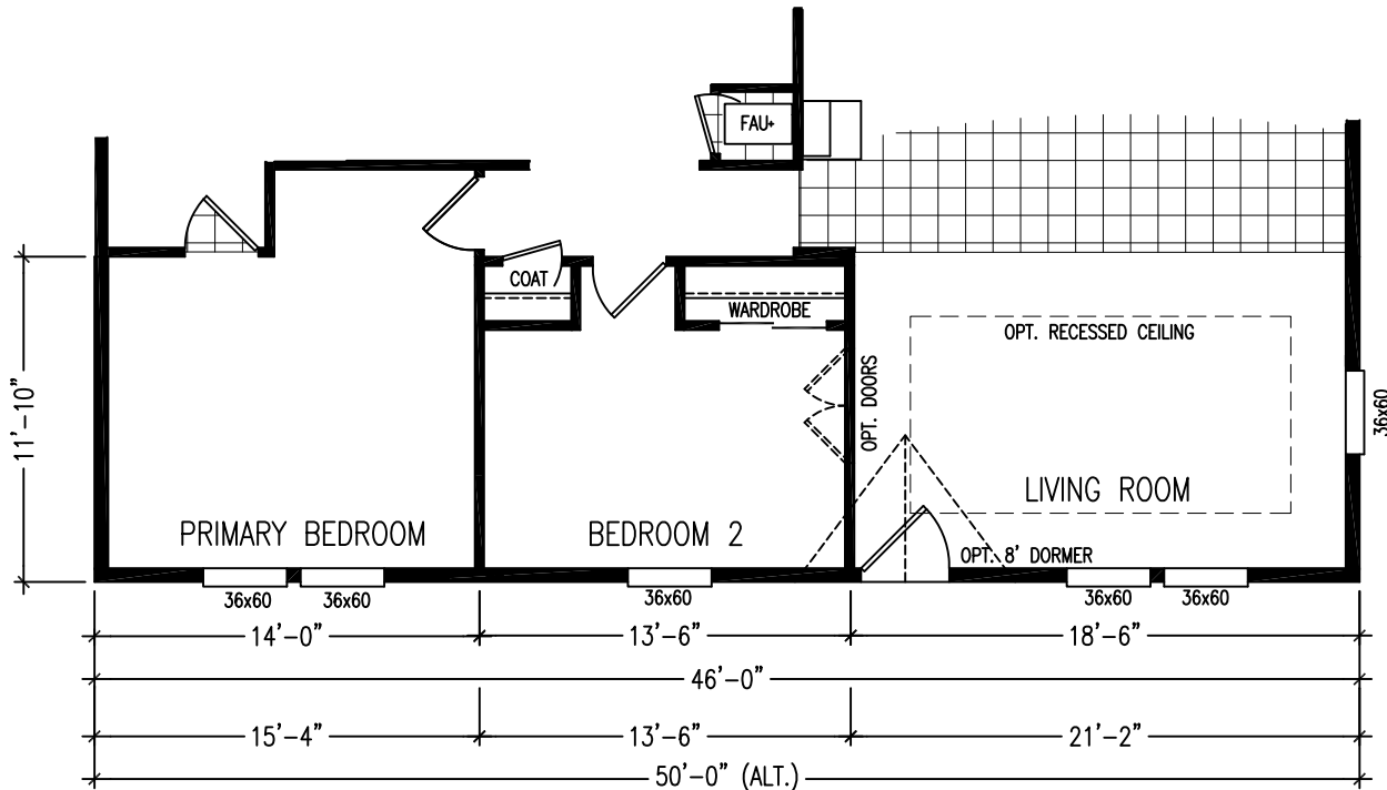
OPTIONAL 2-BEDROOM LAYOUT
